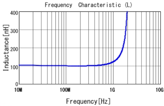
■ LQW18ASR10G0C L
