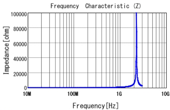
■ LQW18ASR10G0C |Z|
