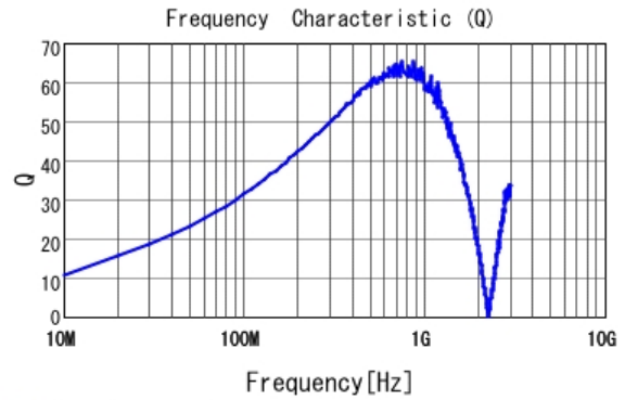
■ LQW18ASR10G0C Q
