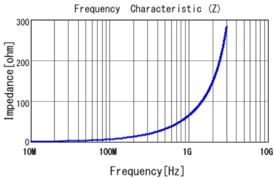
■ LQW18AS10NG0C |Z|
