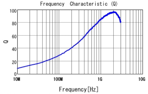
■ LQW18AS10NG0C Q
