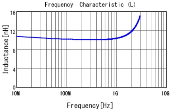
■ LQW18AS10NG0C L
