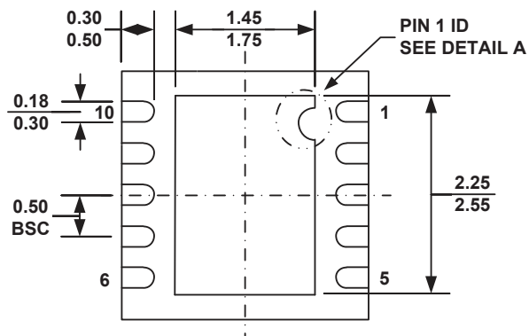
3mm x 3mm QFN10
