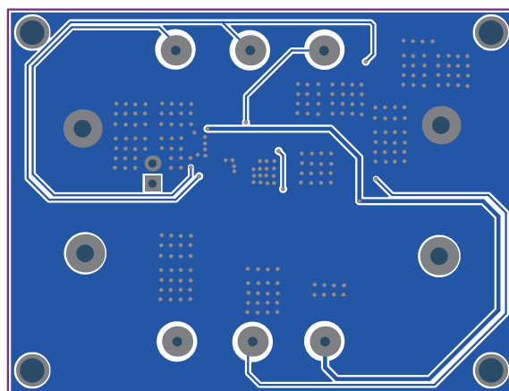
Figure3: Bottom Layer
