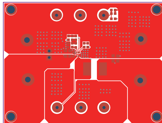
Figure2: Top Layer
