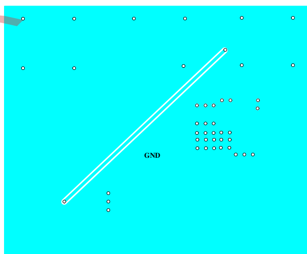
Inner2 Layer
