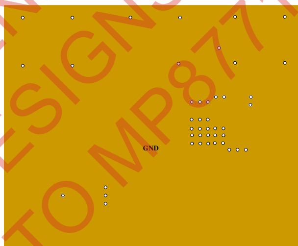
Inner1 Layer
