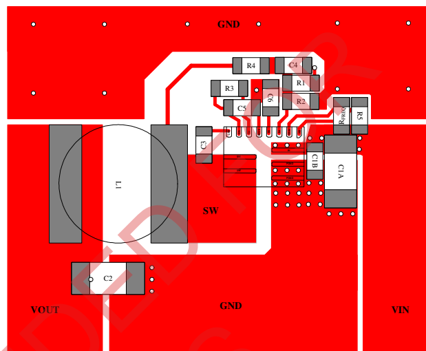
Top Layer
