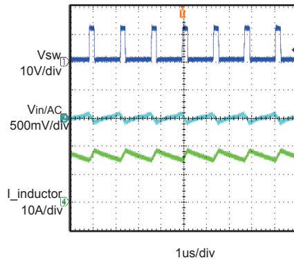
Input Ripple
