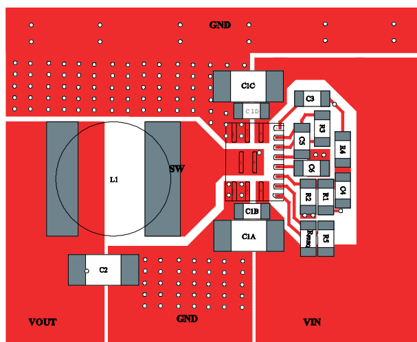
Top Layer
