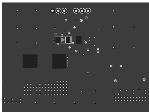
Bottom Layer
