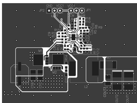
Top Layer
