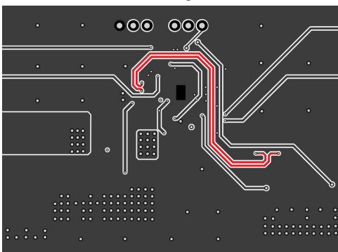
Inner Layer 2
