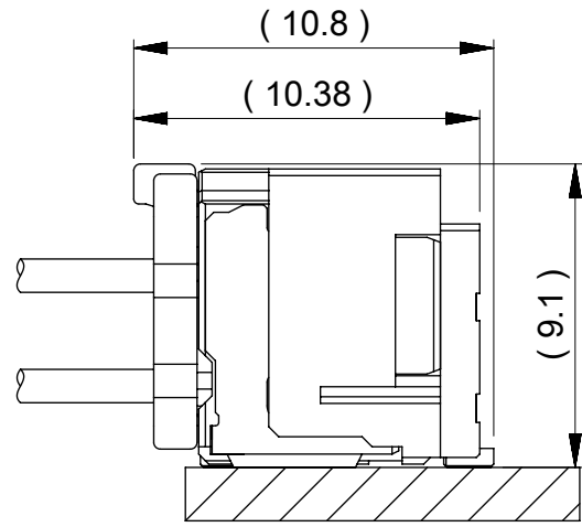
嵌合状態図 MATED CONNECTORS
