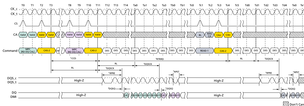
Figure 130: Read DQ Calibration Training Timing: Read DQ Calibration to Read DQ Calibration/Read
