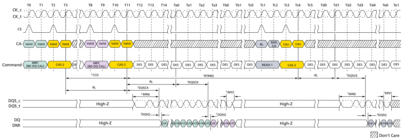
Figure 106: Read DQ Calibration Training Timing: Read DQ Calibration to Read DQ Calibration/Read
