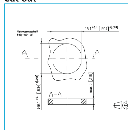
Einbauausschnitt Cut out
