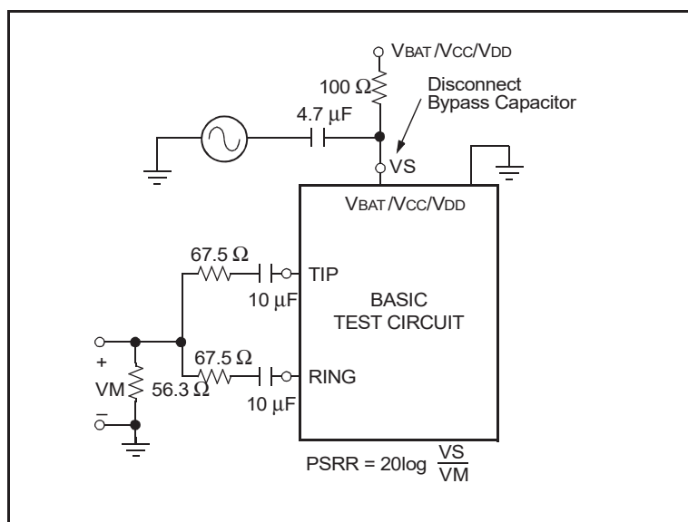
Figure 7-3. Longitudinal PSRR
