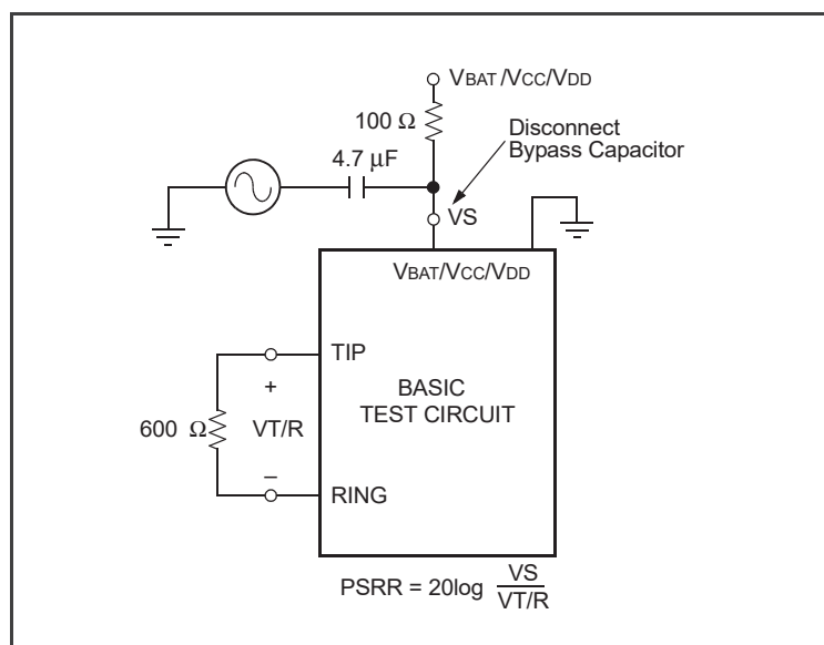
Figure 7-3. Longitudinal PSRR
