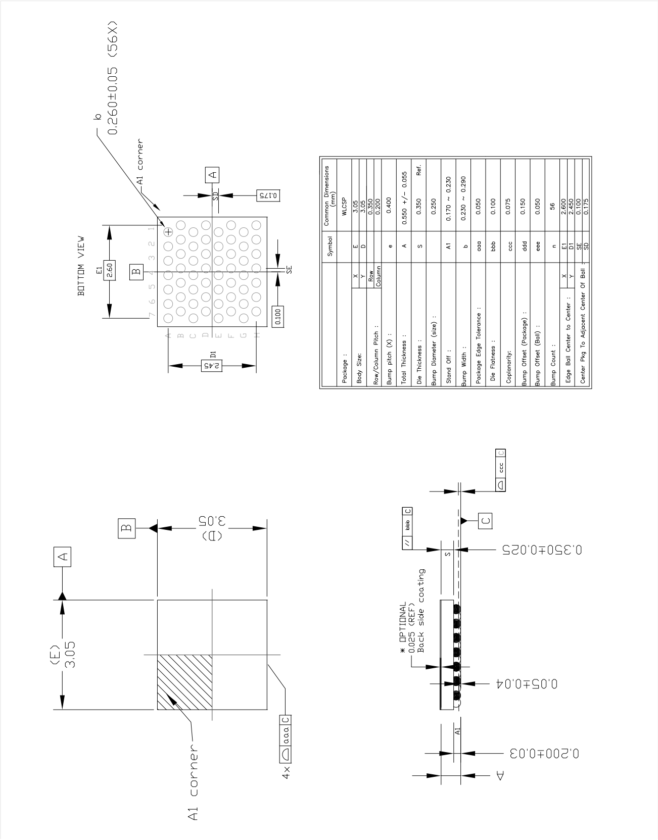
Figure 47 • 56-Ball WLCSP
