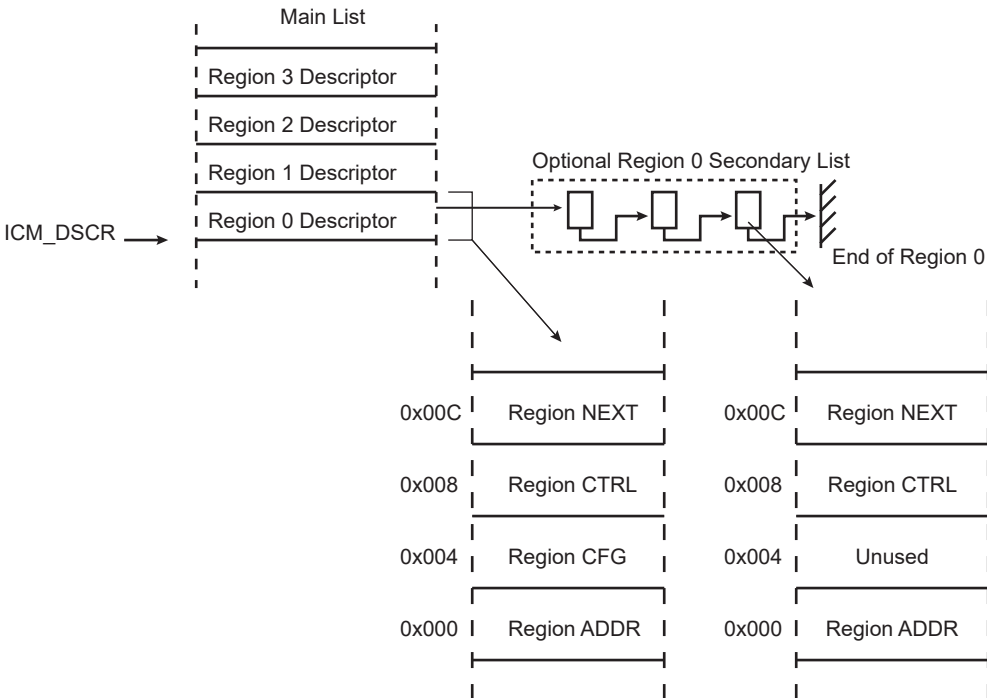
Figure 55-4. Region Descriptor
