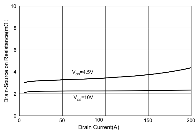
Fig.4 - R_{DS(ON)} - I_D
