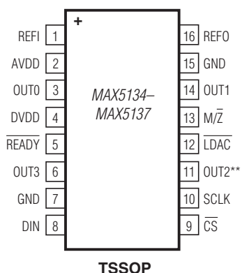
TSSOP
