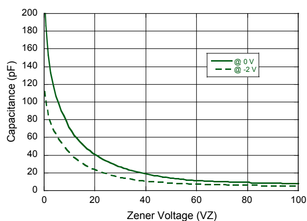
Capacitance vs. Zener Voltage
