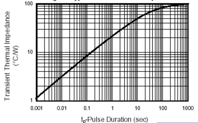
Fig. 8 - Typ. Transient Thermal Impedance
