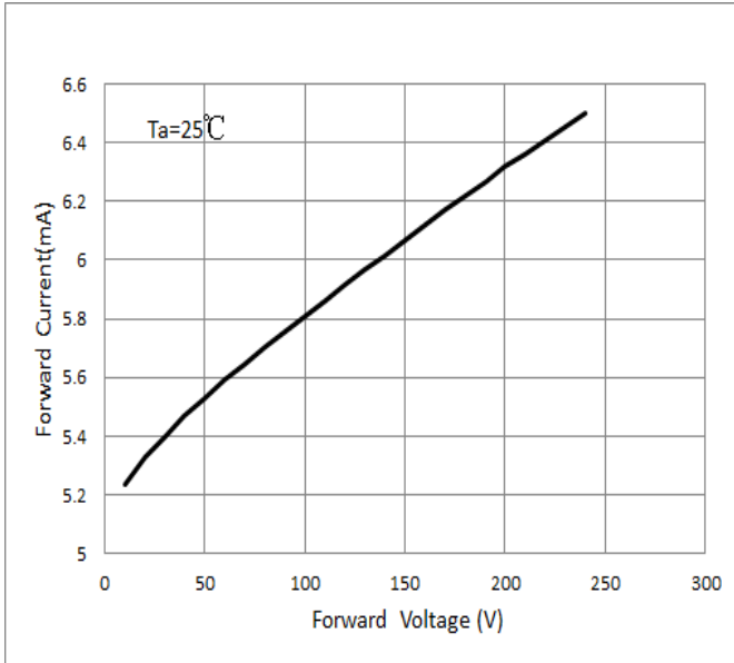
V_f ----- I_f
