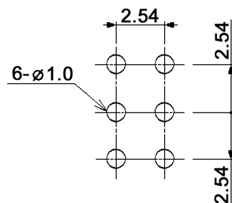
P.C. LAYOUT
