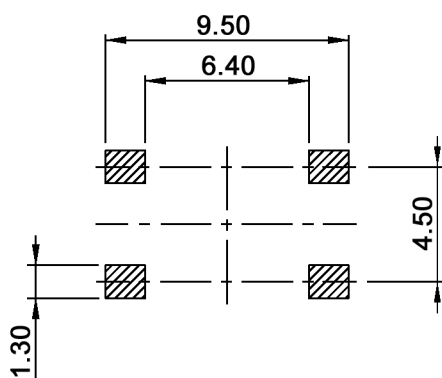
P.C.B. LAYOUT
