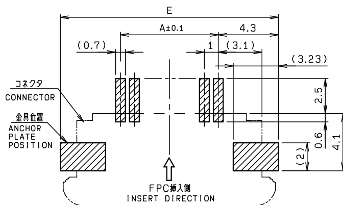
取付け基板寸法 (コネクタ搭載側) MOUNTING LAYOUT
