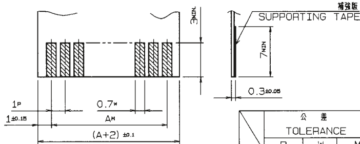
補強板
