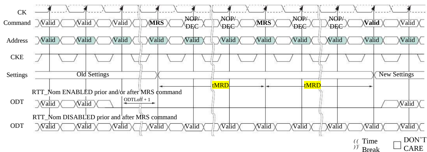
Figure2.3.1a tMRD Timing
