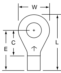
M10-14R/S Stud Size 1/4 Wire Range 12-10
