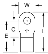
M10-4R/S Stud Size 4 Wire Range 12-10
