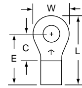
M10-8R Stud Size 8 Wire Range 12-10
