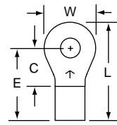
M10-6R Stud Size 6 Wire Range 12-10
