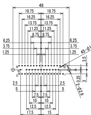
PD-1645BA(10)
