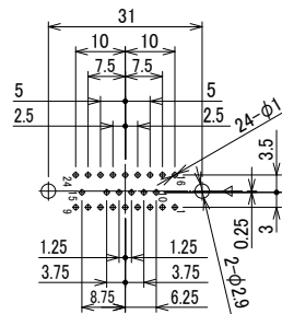
PD-1624BA(09)
