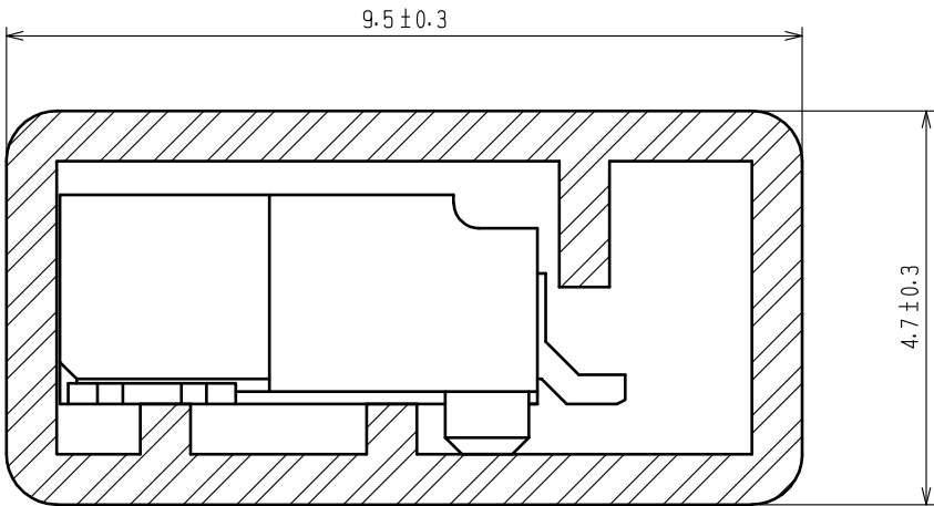
A-A ( 10 : 1 )
