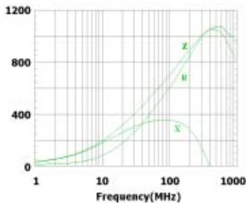
GBG160808GZA601N
