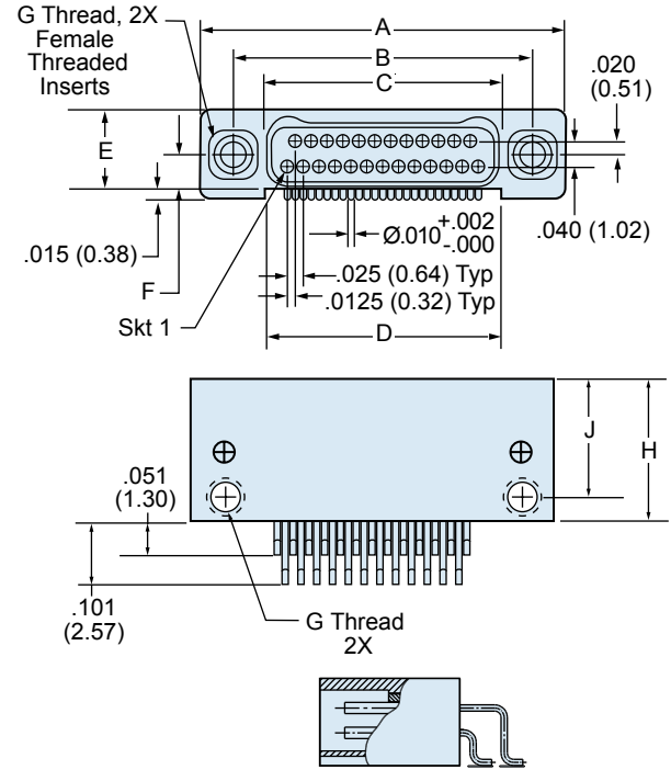
891-013 Receptacle (Socket) Connectors
