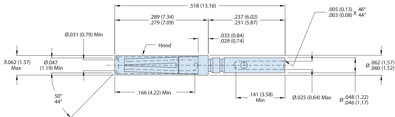
857-218-22-30 - DIMENSIONS
