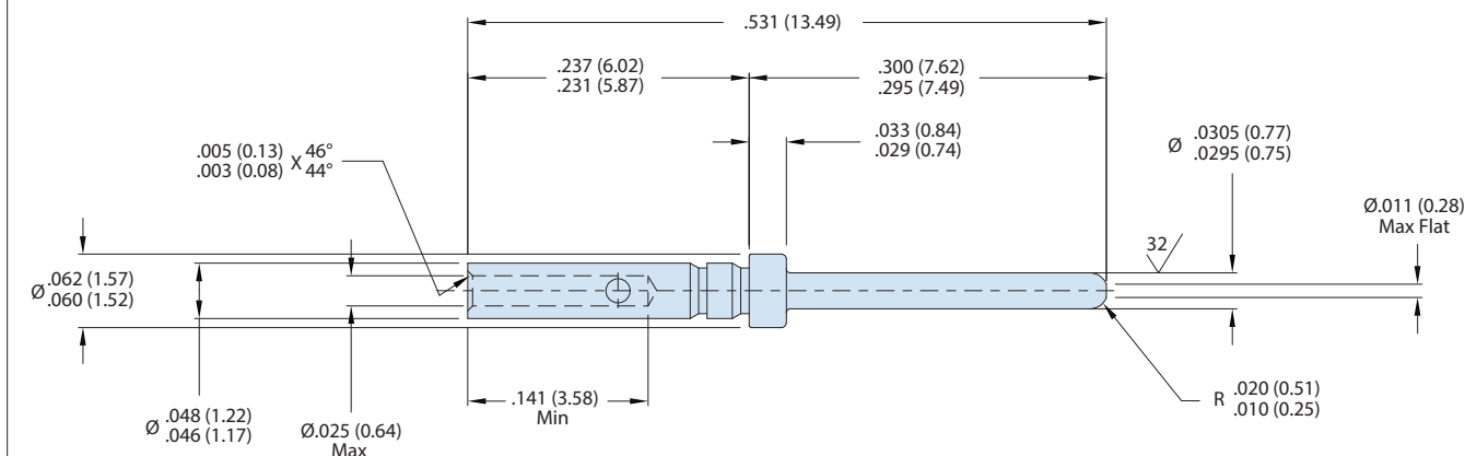
857-217-22-30 - DIMENSIONS
