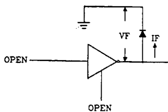
7. V_F
