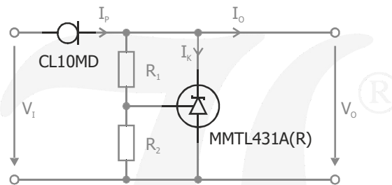
Fig. 3 Spannungsversorgung mit geringem Bauteilbedarf für \mu Controller und andere Schaltungen mit niedrigem Eingangsstrom
