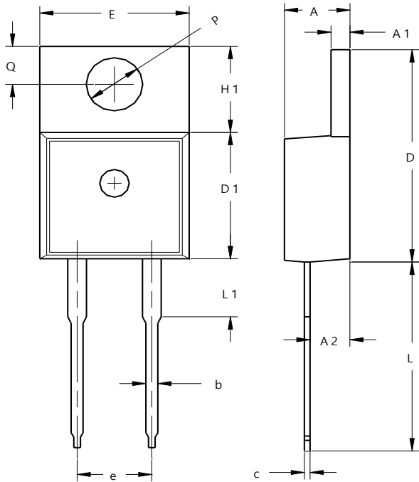
TO220AC (Type WX)
