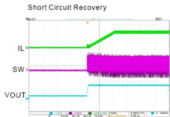
V_{in}=3.3\text{V} , V_o=1.2\text{V} , I_o=3.5\text{A}
