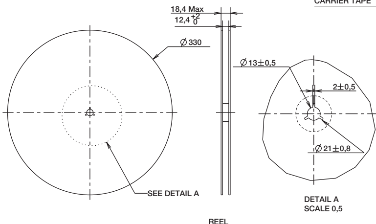
REEL
