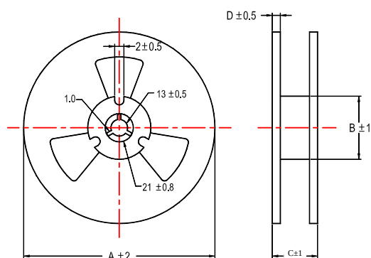
Reel Dimensions
