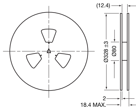
REEL DIMENSIONS
