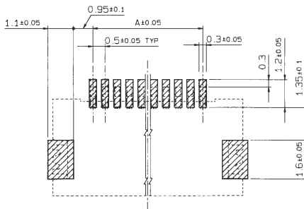
基板配付寸法 MOUNTING LAYOUT
