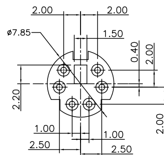
DETAIL B 1:1
