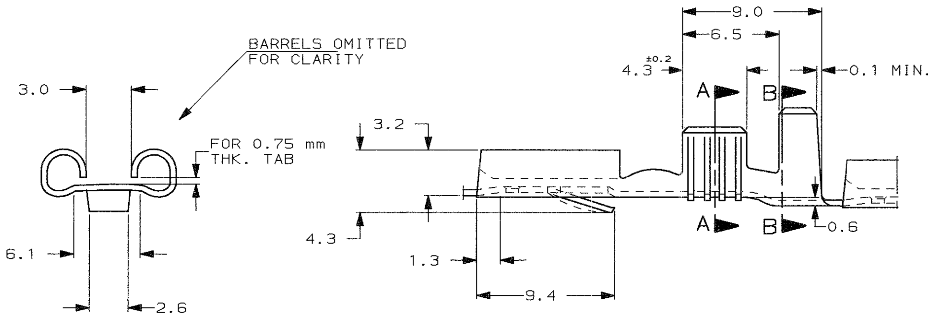
SEZIONE A-A (SECTION A-A)
