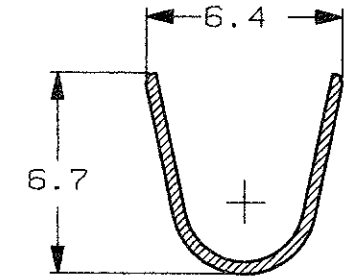
SEZIONE B-B (SECTION B-B)
