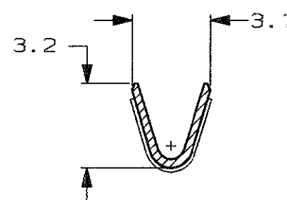
SEZIONE A-A (SECTION A-A)
