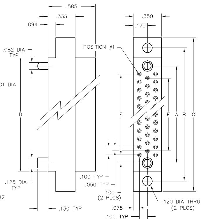
RECEPTACLE
