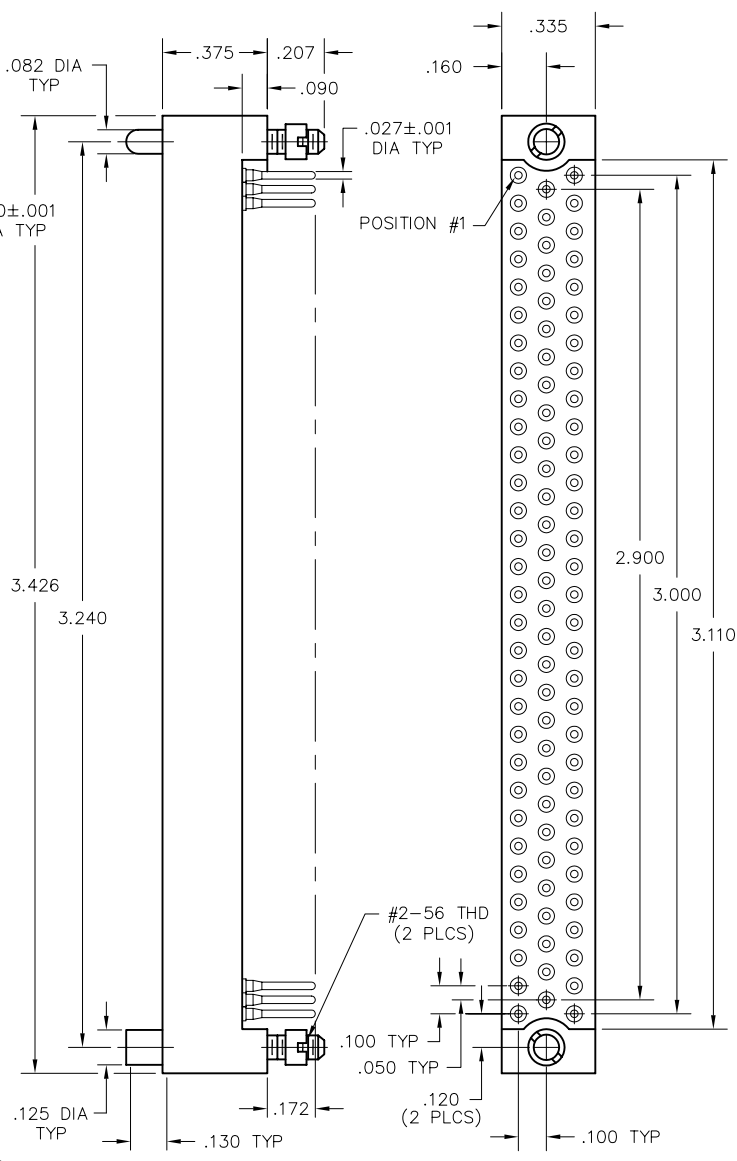
RECEPTACLE
