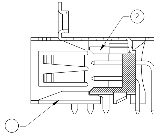
SECTION A-A SCALE 4:1
