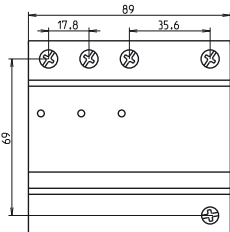
OVR T1+2 3N 15-255-7
