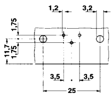
PSC 1,5/3-M
