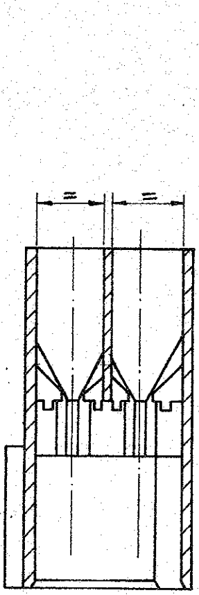
SEC. A-A (SCALE 2:1)
